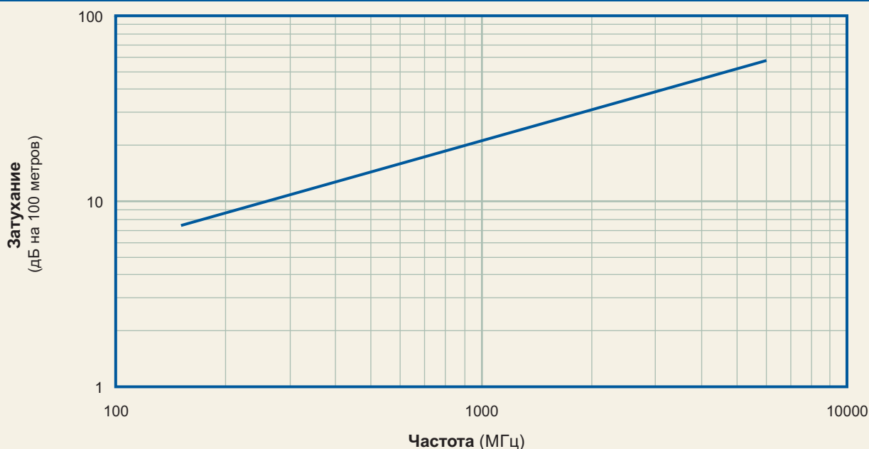
Типовое затухание 5D-FB PVC SCALAR
